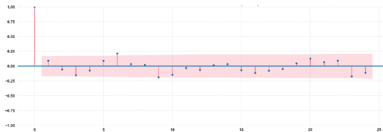
Figura 8.17: ACF de Residuos del modelo Holt-Winters
