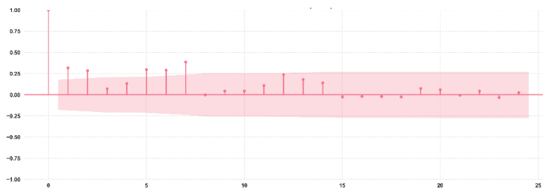
Figura 8.18: ACF de Residuos del modelo Random Forest
